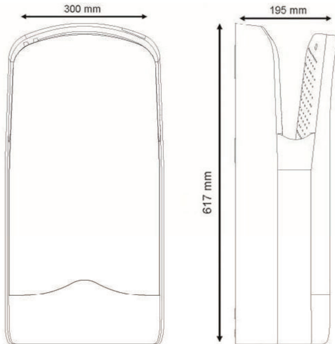
Dimensiones en mm.
